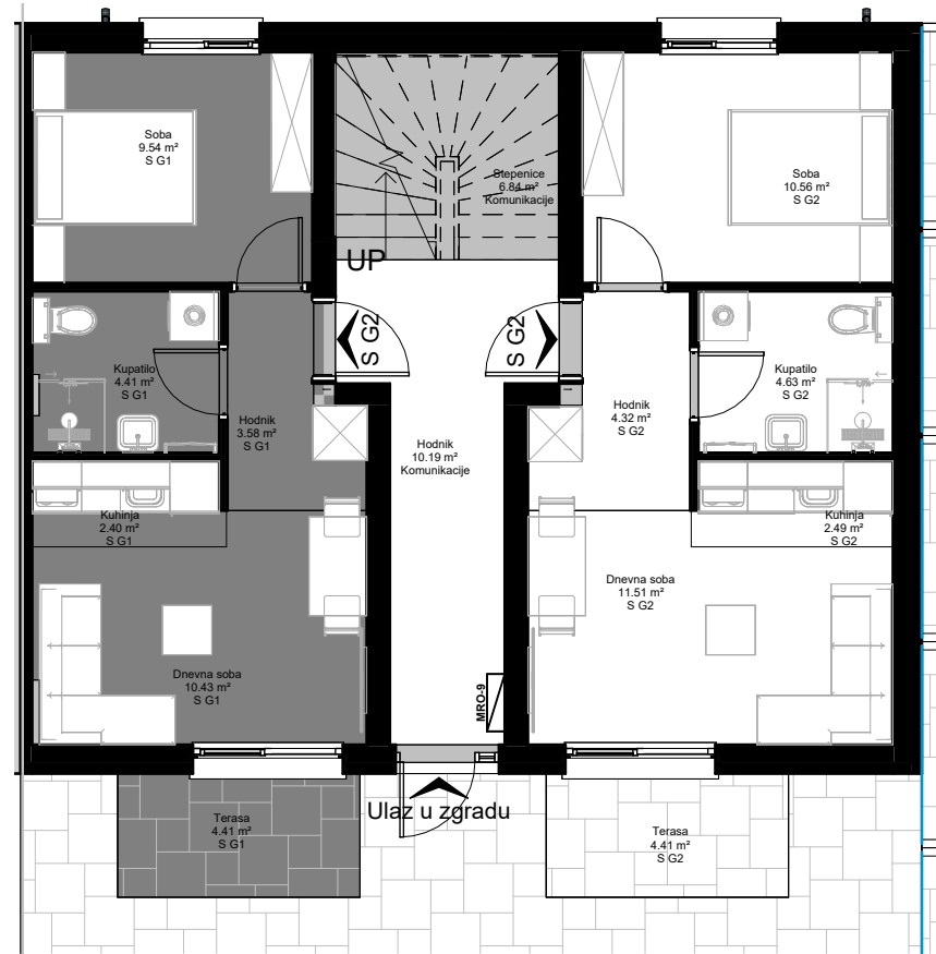
1 C02 - Prizemlje - Položaj stana S G1 na osnovi 1 : 100
